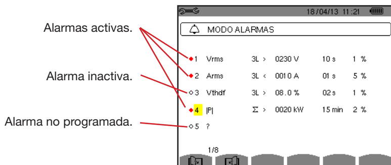
Figura 34: el menú Modo alarma
