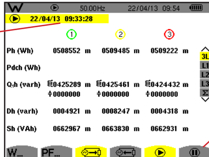
Figura 117: la pantalla de inicio de la medición de energía en Wh
