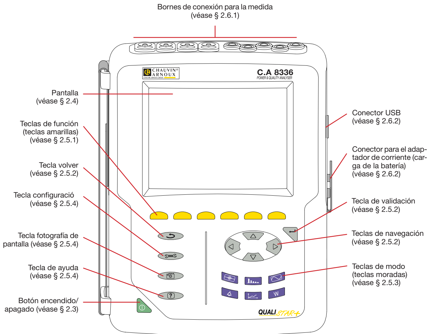
Figura 1: vista general del Qualistar+
