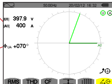
Figura 84: la pantalla de visualización del diagrama de Fresnel en Bifásico de 2 hilos
